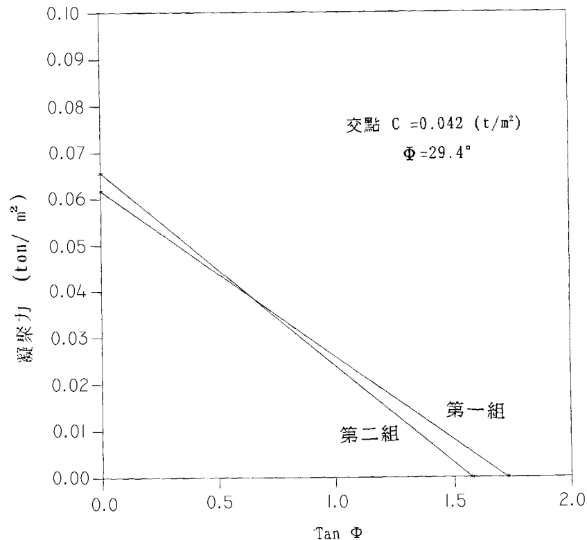
圖 4 逆算法之 C 對 \tan \phi 之關係圖
