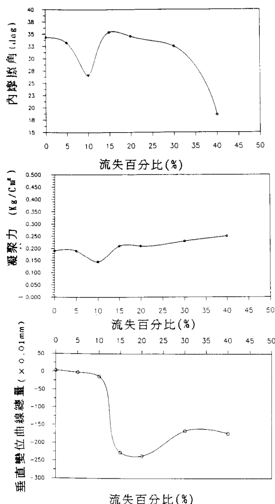
圖 1 直剪試驗結果之凝聚力、內摩擦角與垂直變位曲線總量之綜合分析圖
