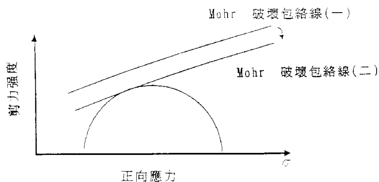
圖 3 土壤強度降低，包絡線下降示意圖
