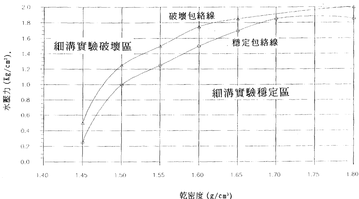
圖 2 乾密度、水壓力穩定與破壞包絡線
