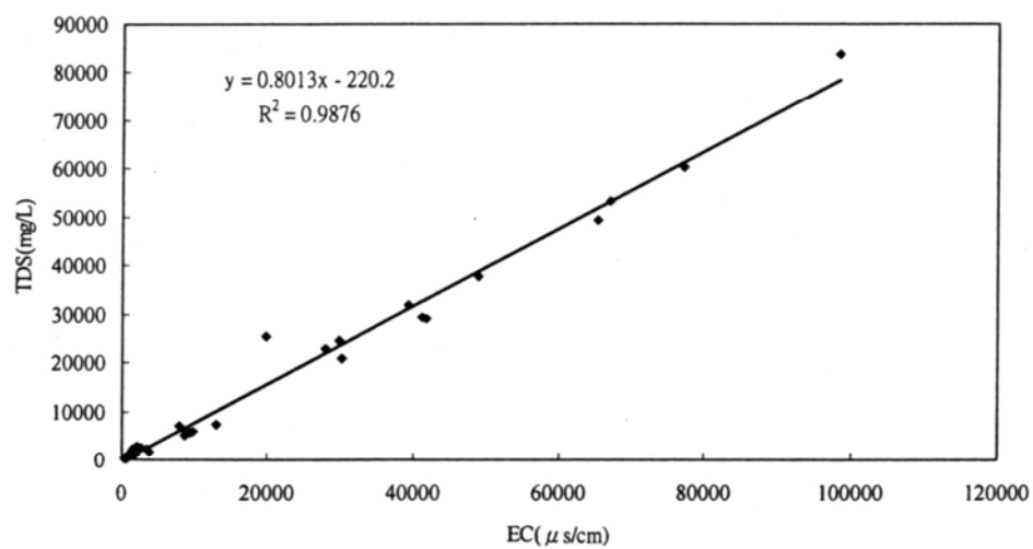
圖 2 嘉南平原地下水水質電導度(EC)與總溶解固體物(TDS)關係
