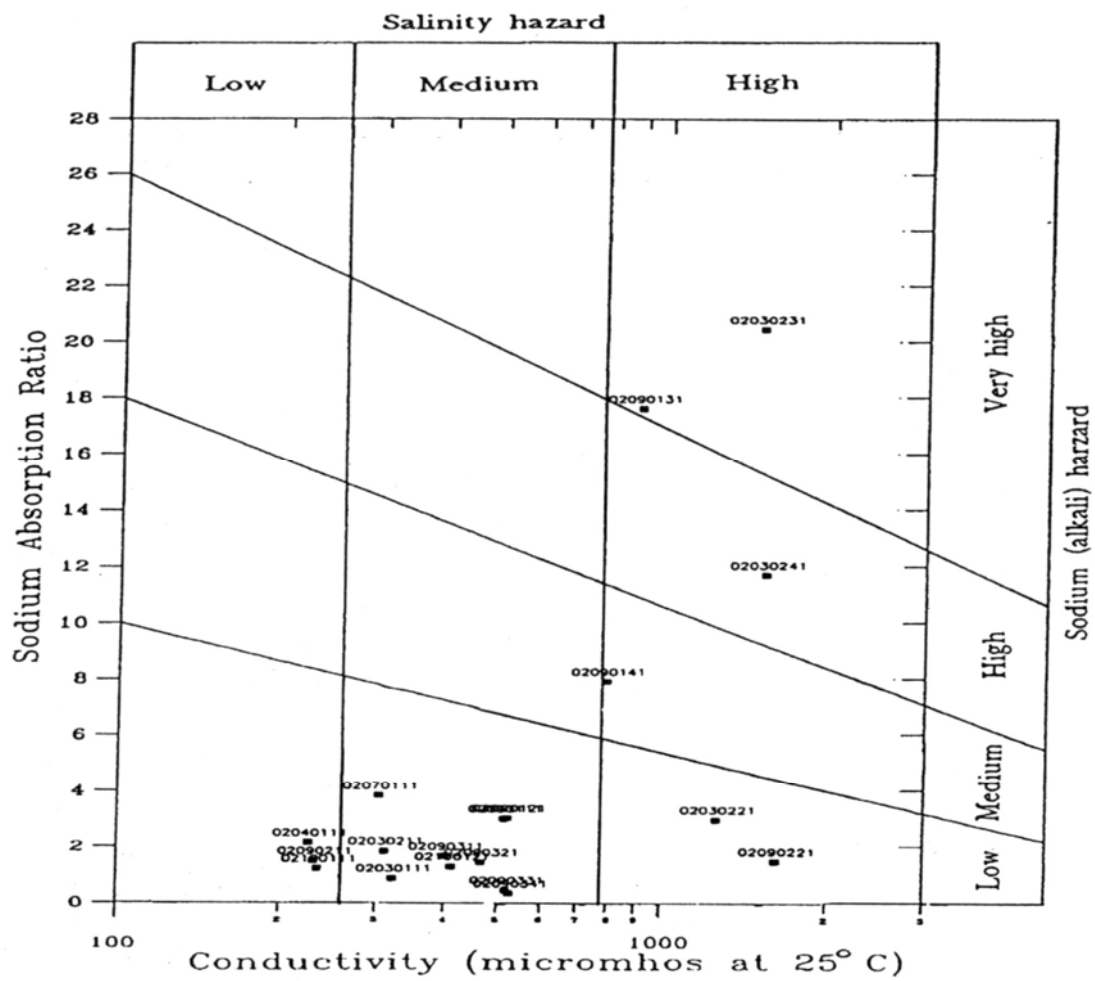
圖 3 蘭陽平原八十九年度 SAR 與電導度關係顯示對土壤的影響
