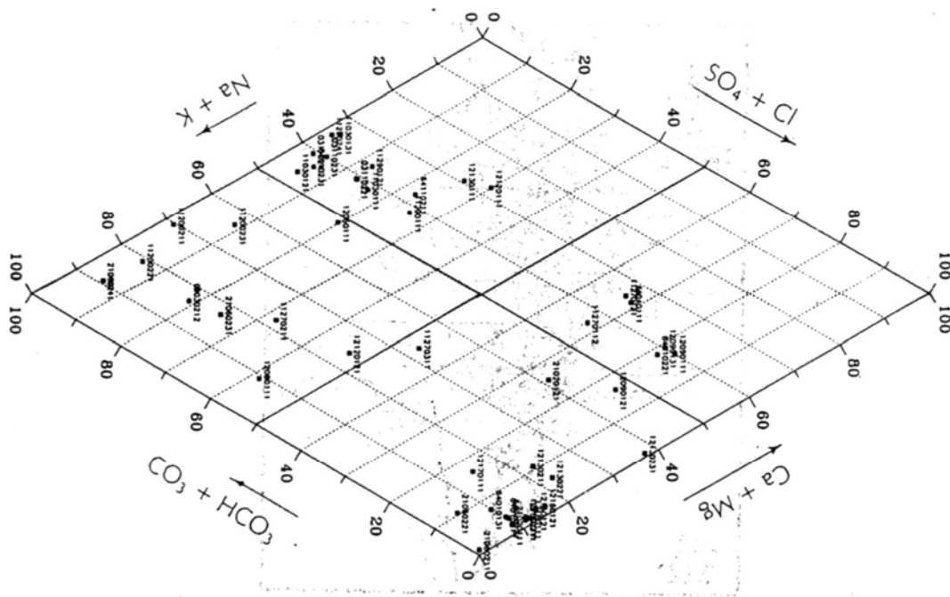
圖 6 嘉南平原地區地下水水質菱形圖(89 年度資料)
