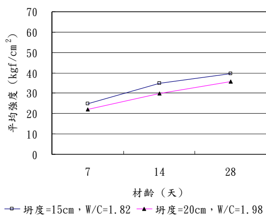
圖 22 室內強度試驗結果
