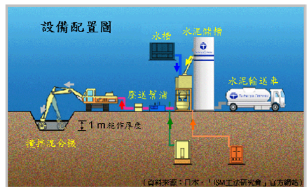
圖 6「ISM 工法」現場設備配置圖
