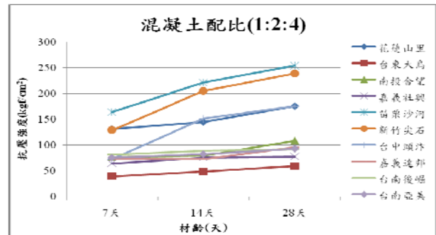
圖 19 10 處取樣地點配比(1:2:4)之抗壓試驗比較
