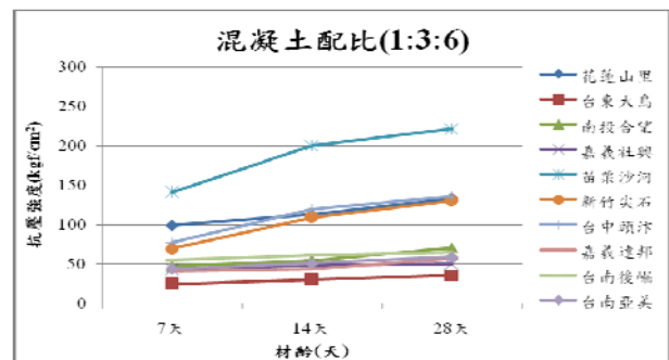
圖 20 10 處取樣地點配比(1:3:6)之抗壓試驗比較
