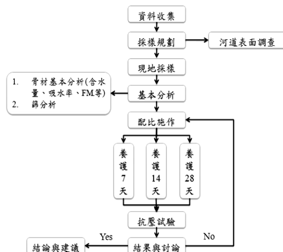
圖 7 配比試驗流程圖
