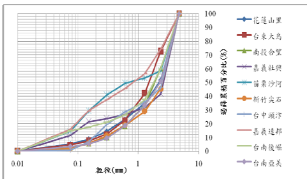
圖 18 10 處取樣地點細骨材粒徑分佈曲線比較
