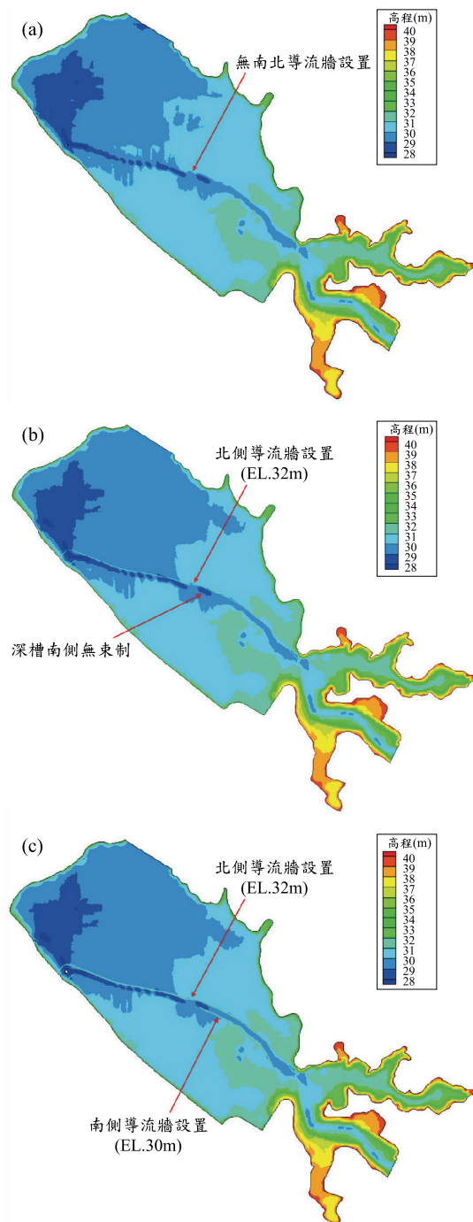
圖 2 阿公店水庫庫區設置導流牆 (a) 無設置、(b) 北側導流牆設置、(c) 南北側導流牆設置
