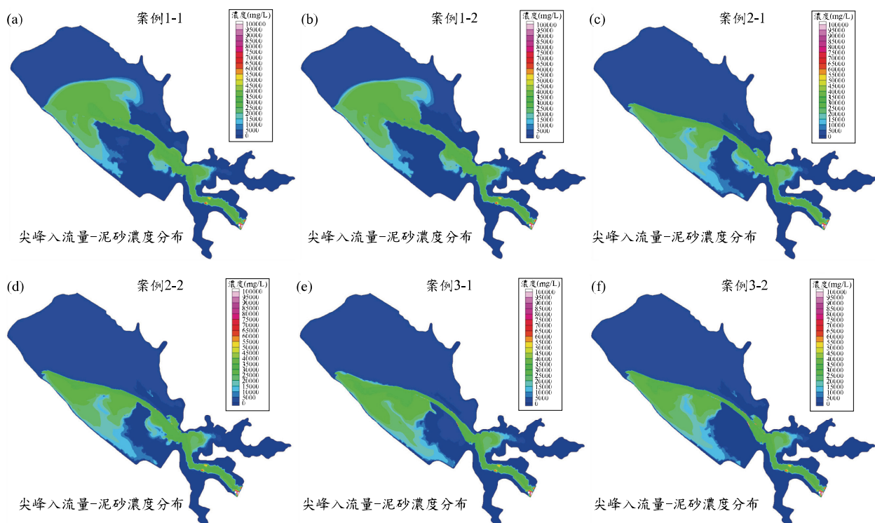
圖 6 尖峰入流量時庫區濃度分布 (a) 無冲刷槽導流牆案例 1-1、(b) 無冲刷槽導流牆案例 1-2、(c) 冲刷槽北側佈置導流牆案例 2-1、(d) 冲刷槽北側佈置導流牆案例 2-2、(e) 冲刷槽南北側皆佈置導流牆案例 3-1、(f) 冲刷槽南北側皆佈置導流牆案例 3-2
