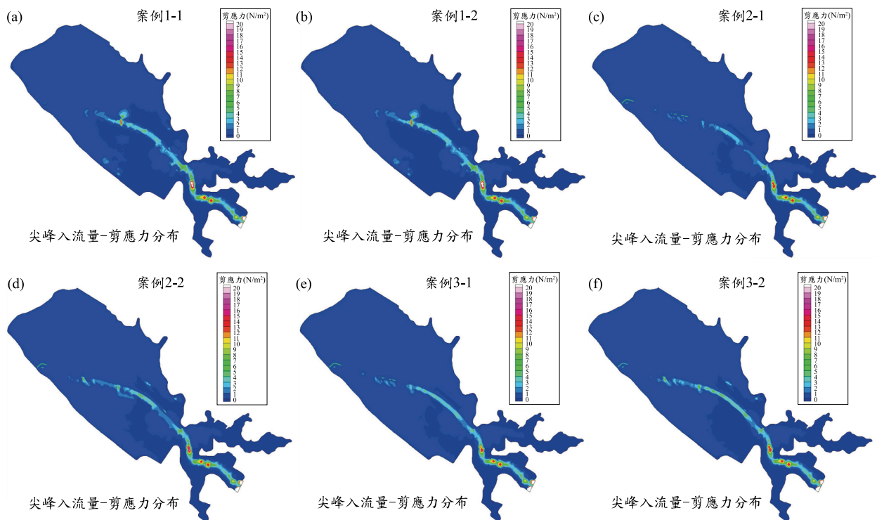
圖 7 尖峰入流量時庫區剪力分布 (a) 無冲刷槽導流牆案例 1-1、(b) 無冲刷槽導流牆案例 1-2、(c) 冲刷槽北側佈置導流牆案例 2-1、(d) 冲刷槽北側佈置導流牆案例 2-2、(e) 冲刷槽南北側皆佈置導流牆案例 3-1、(f) 冲刷槽南北側皆佈置導流牆案例 3-2
