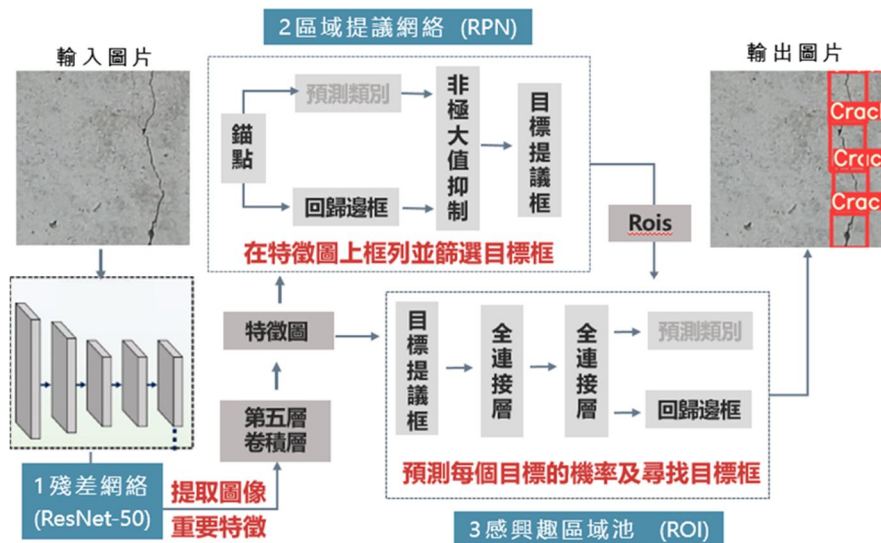
圖 4 本研究 Faster R-CNN 實驗模型架構圖
