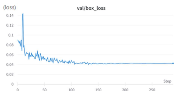
圖 6 驗證集 (validation dataset) loss 曲線圖
