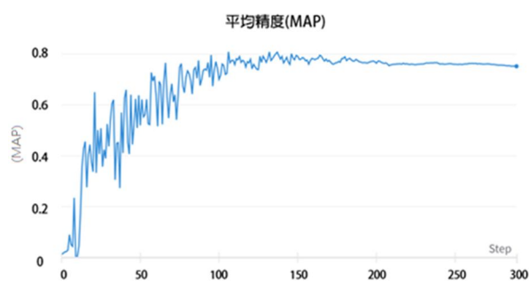
圖 9 實驗成果平均精度 (MAP) 圖
