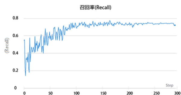
圖 8 實驗成果召回率 (Recall) 圖
